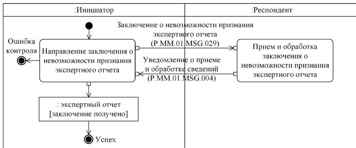
Рис. 15. Схема выполнения транзакции общего процесса «Направление заключения о невозможности признания экспертного отчета» (P.MM.01.TRN.020)
