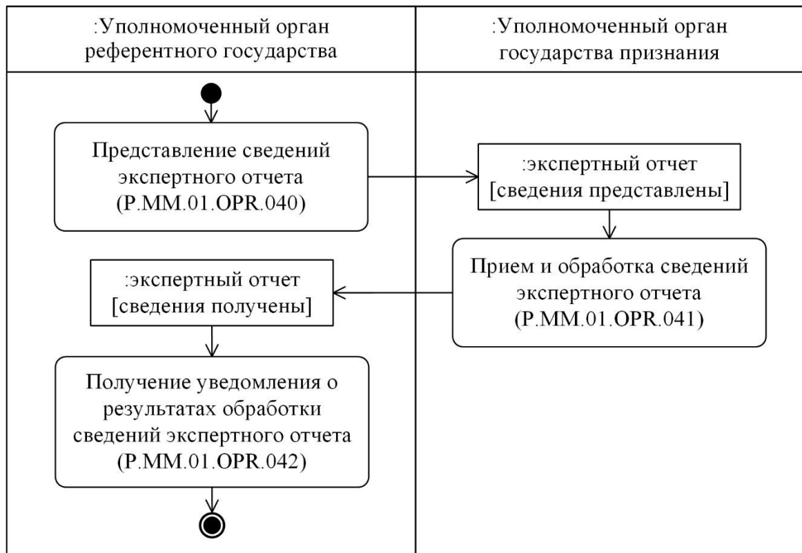
Рис. 29. Схема выполнения процедуры «Направление экспертного отчета» (P.MM.01.PRC.014)
