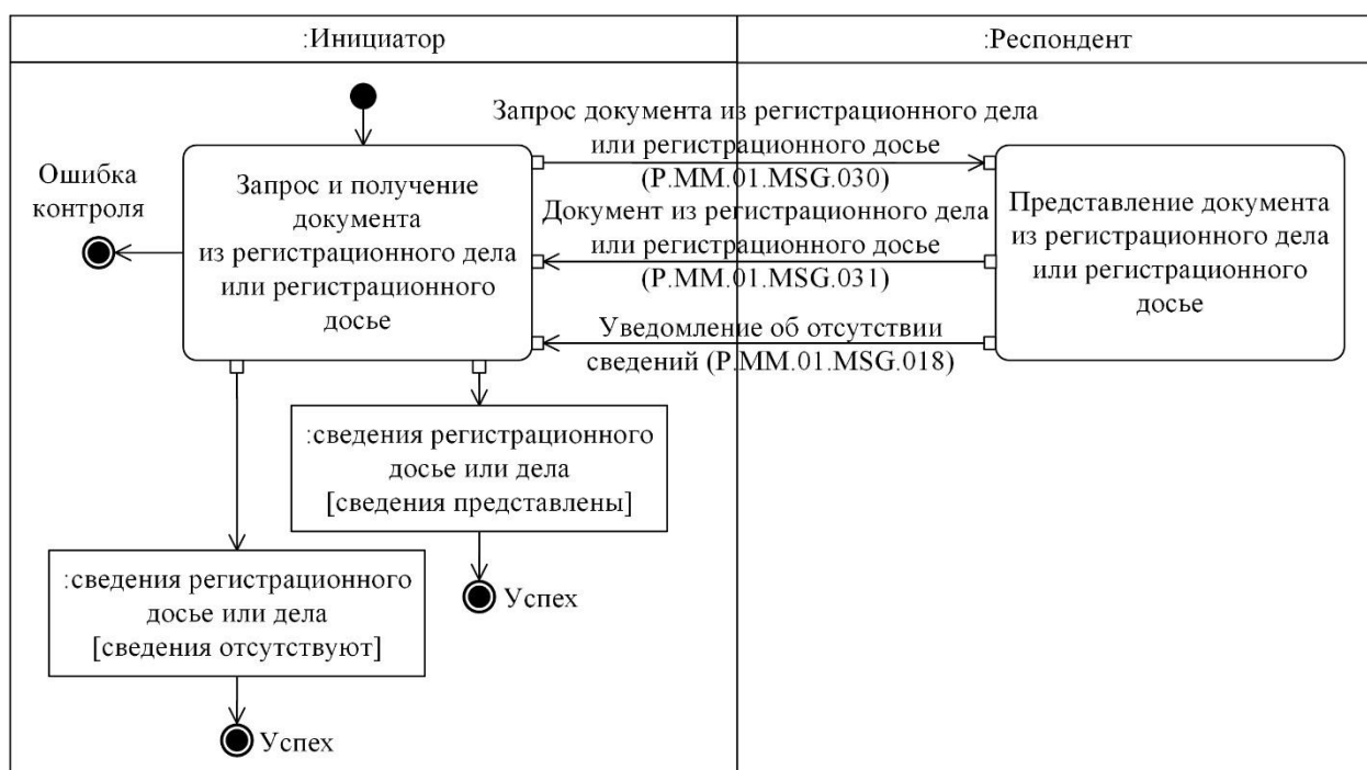
Рис. 16. Схема выполнения транзакции общего процесса «Получение Комиссией документа из регистрационного дела или регистрационного досье» (P.MM.01.TRN.021)
