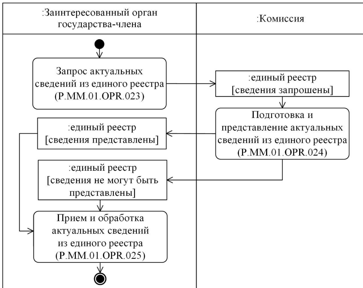
Рис. 17. Схема выполнения процедуры «Получение актуальных сведений из единого реестра» (P.MM.01.PRC.008)
