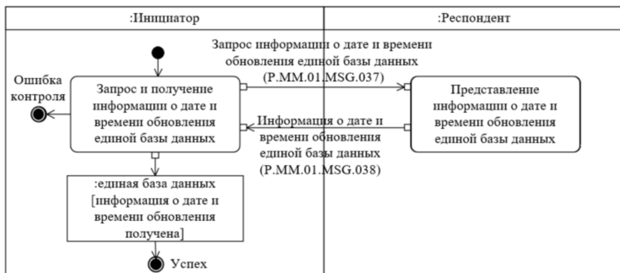
Рис.21. Схема выполнения транзакции общего процесса «Получение информации о дате и времени обновления единой базы данных» (P.MM.01.TRN.027)
