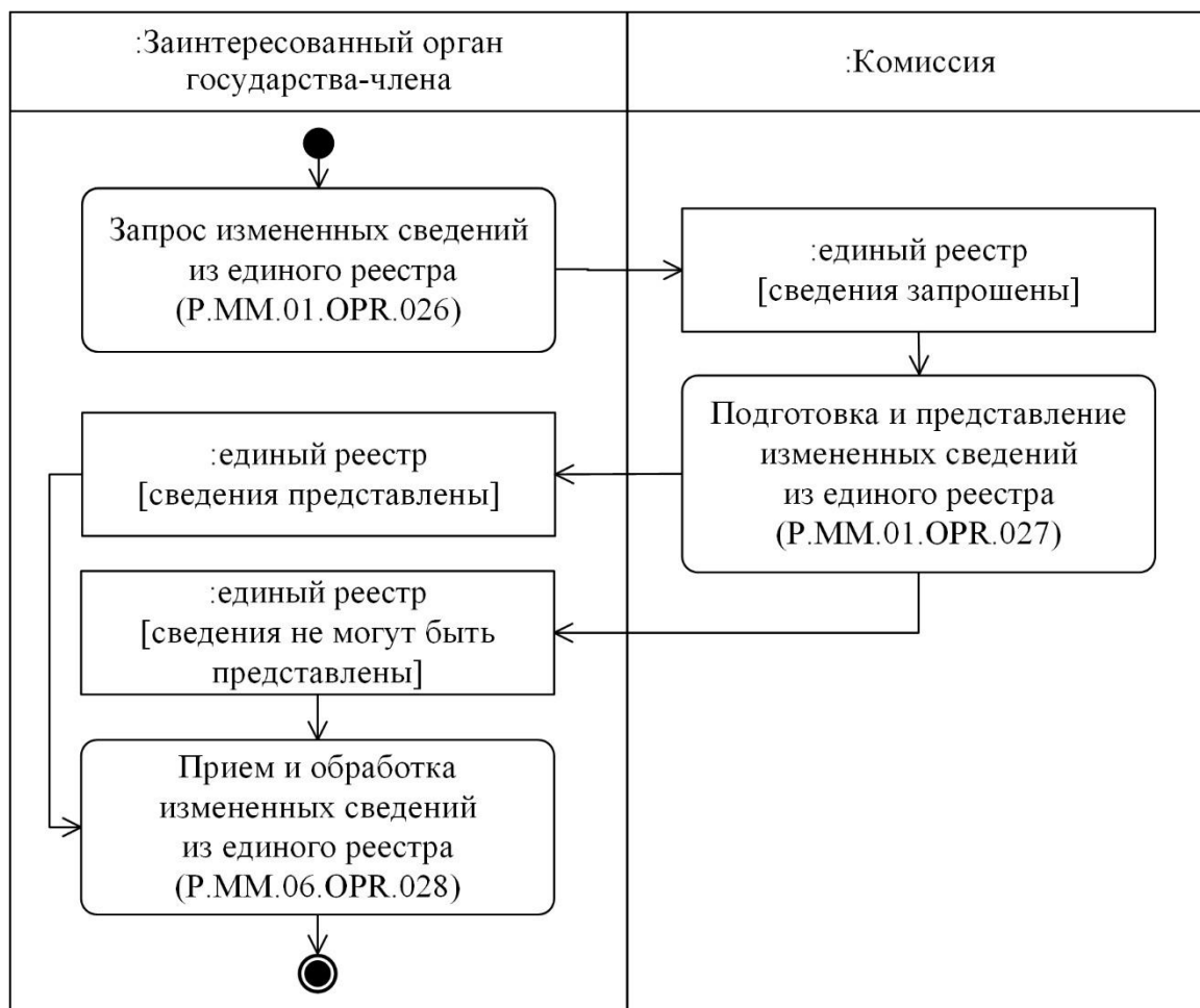
Рис. 18. Схема выполнения процедуры «Получение измененных сведений из единого реестра» (P.MM.01.PRC.009)
