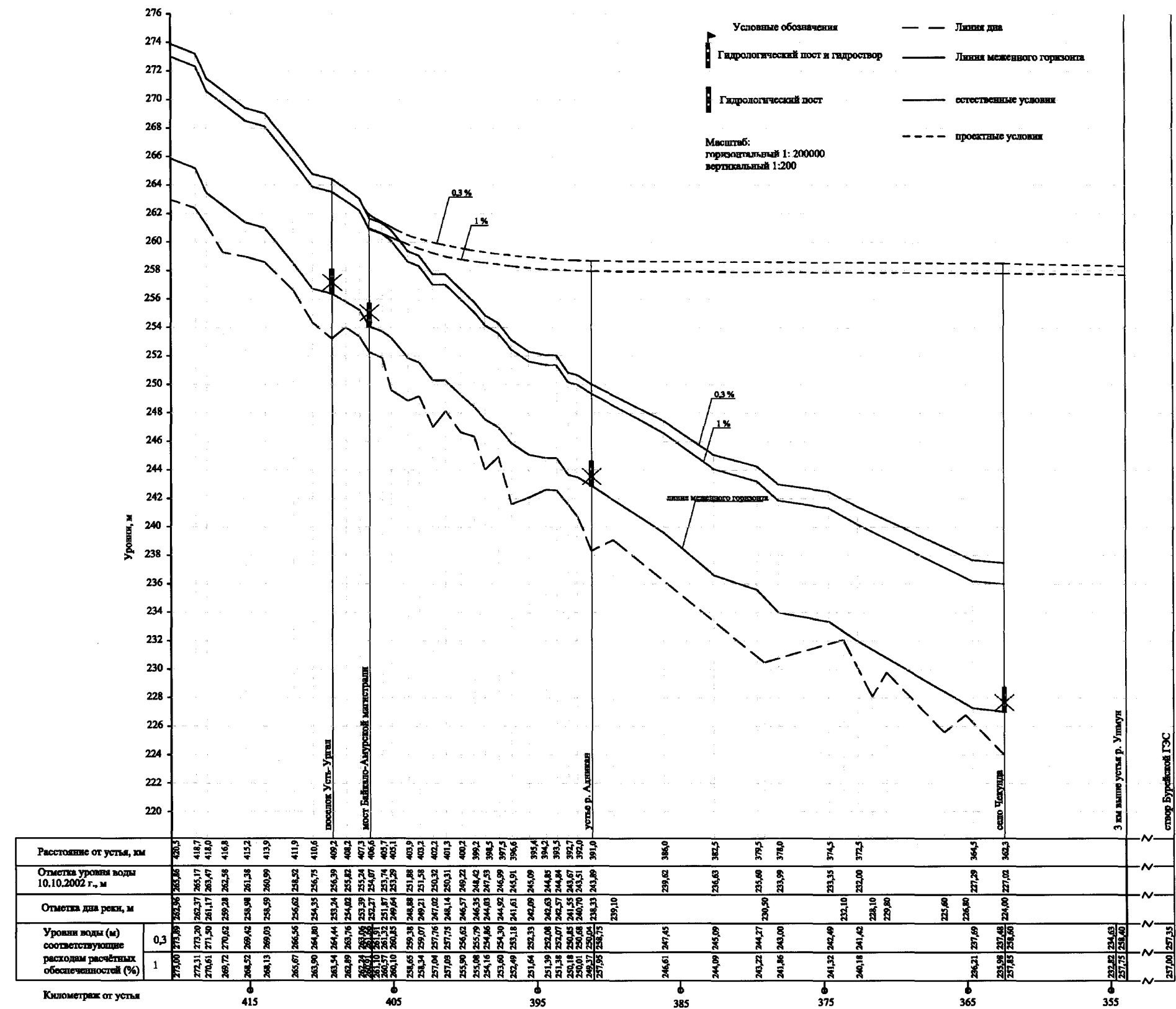
Кривые свободной поверхности р. Буреи в естественных и проектных условиях на участке от 3 км выше устья р. Ушмун до поселка Ургал при прохождении дождевых паводков расчетных вероятностей превышения
