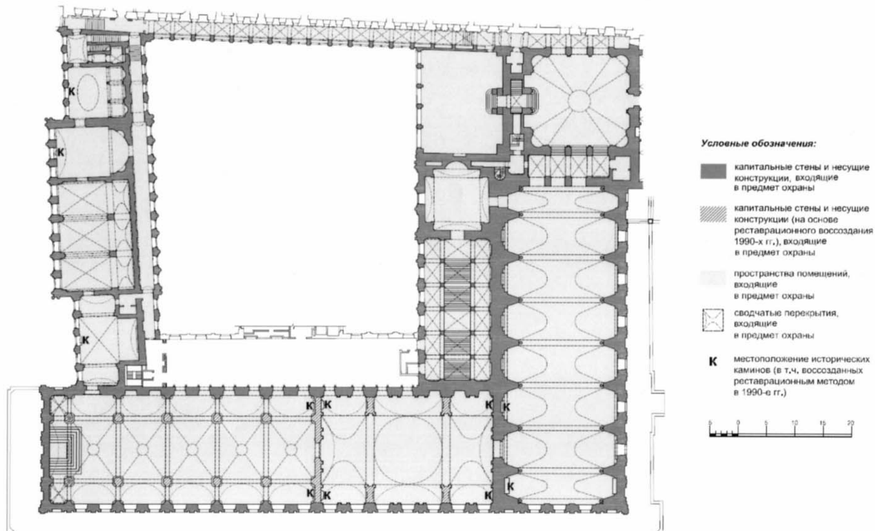
ПЛАН 2-ГО ЭТАЖА
