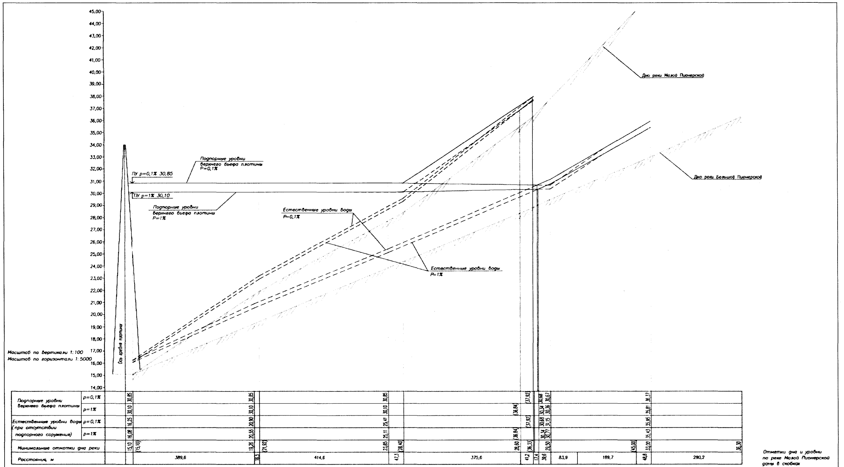
Продольный профиль расчетных кривых свободной поверхности водохранилища и водотоков в верхнем бьефе Пионерского гидроузла при прохождении максимальных расходов воды расчетной обеспеченности
