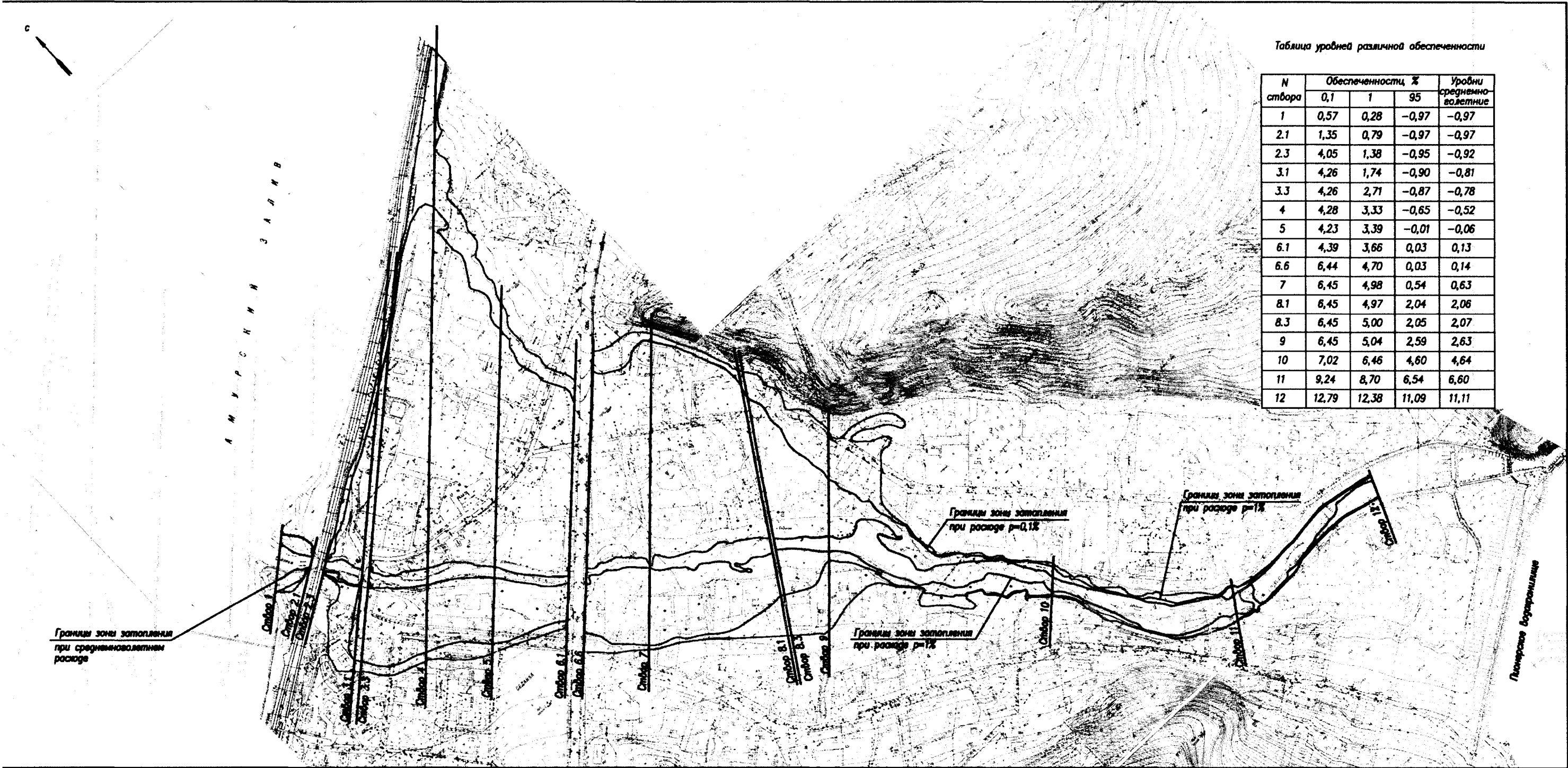
План зон затопления в нижнем бьефе Пионерского водохранилища при прохождении расходов различной обеспеченности
